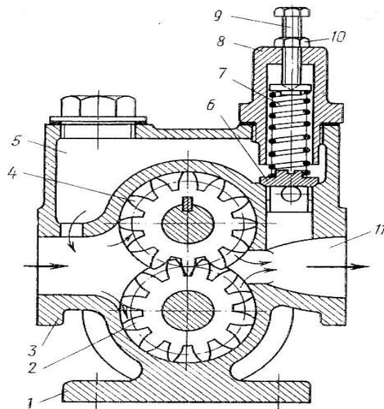
Рисунок 3 – Устройство и схема работы шестерённого насоса с редукционным клапаном:
