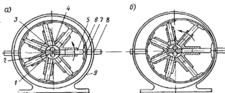
Рисунок 10 – Схема радиально-поршневого насоса: 1 - перемычка; 2,3 - нижняя и верхняя полости насоса; 4 - ротор; 5 - плунжеры; 6 - ползуны; 7 - направляющие кольца; 8 - цапфы; 9 - корпус насоса
