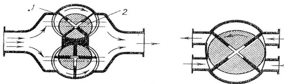
Рисунок 8 – Многопластинчатые насосы: 1 – пластина; 2 – ротор
