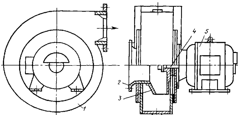
Рис. 3.5. Котельный вентилятор
