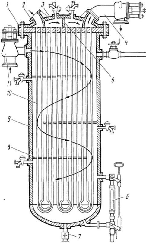
Рис. 3.1. Подогреватель топлива клапан 7. Подогреватель петлевого типа является достаточно надежным теплообменным
