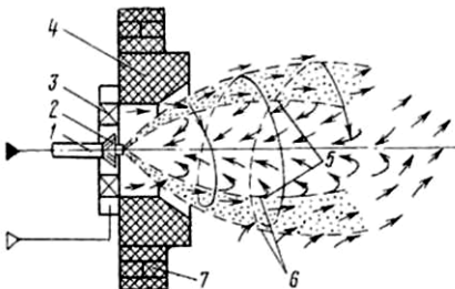
Рис. 3.3. Аэродинамическая структура факела
