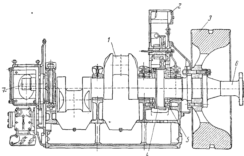
Рис. 7. Коленчатый вал двигателей типа NVD-48 и NVD-36 : 1 — коленчатый вал, 2 — кожух коробки передач, 3 — маховик, 4 — гребень упорного подшипника, 5 — полукольцо, 6 — промежуточный вал, 7 — кривошип привода компрессора и водяных насосов.
