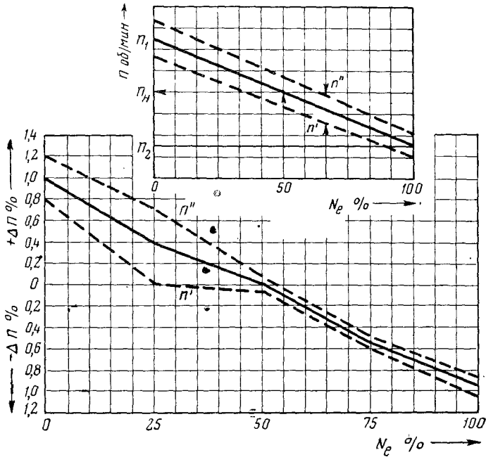
Рис. 63. Регуляторные статические характеристики: вверх — прямолинейная условная основная; вниз — фактическая, снятая при испытании двигателя 7Д12; n'' - n' — зона нечувствительности.
