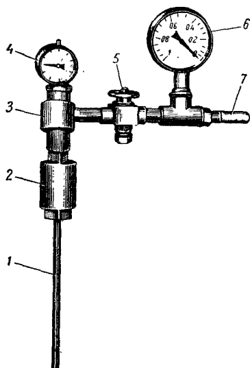
Рис. 102. Прибор для определения зазоров в мотылевом и головном подшипниках:
