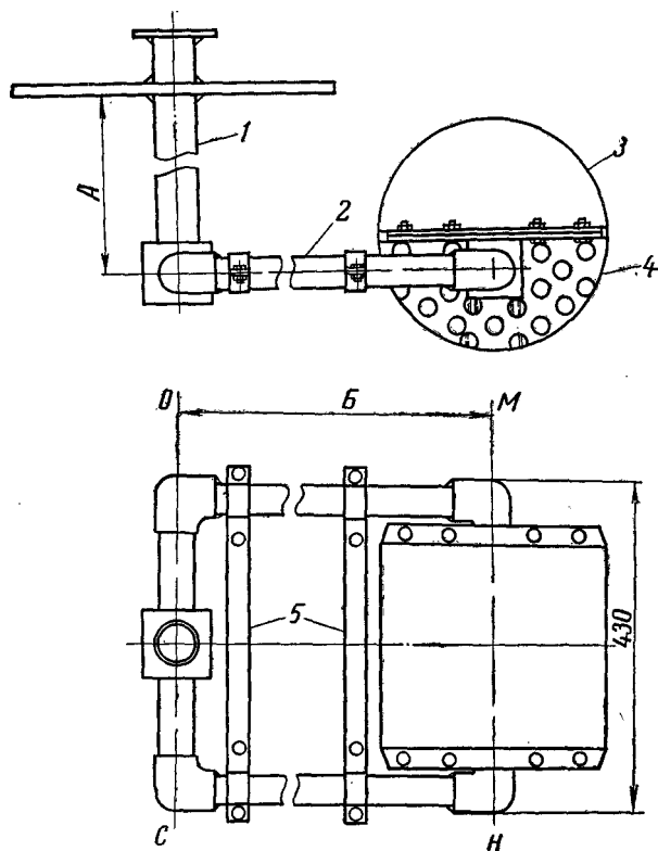
Рис. 120. Поплавковый приемник топлива:
