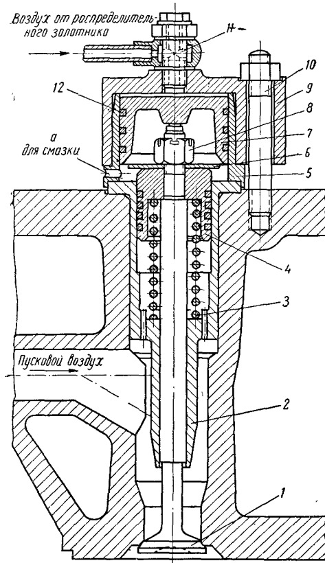
Рис. 35. Пусковой клапан двигателей типа NVD-48 и NVD-36 :
