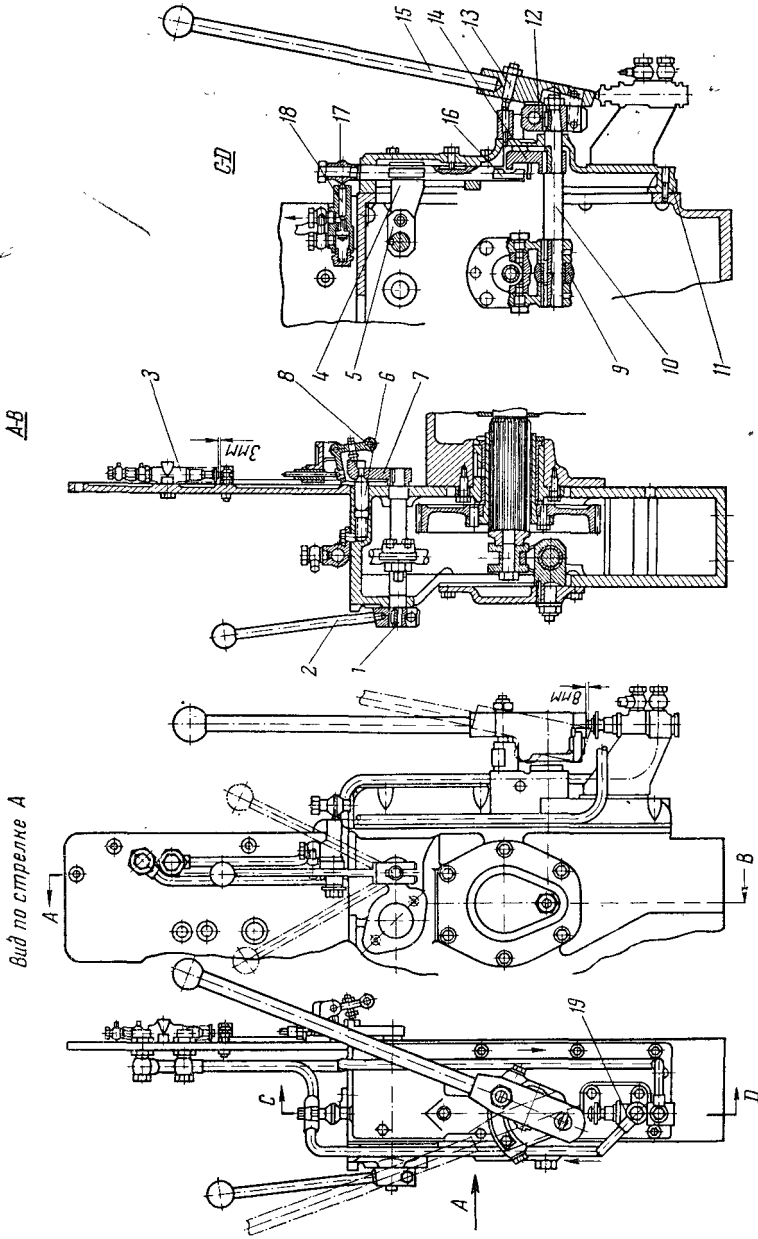
Рис. 42. Пост управления двигателей типа NVD-36:
