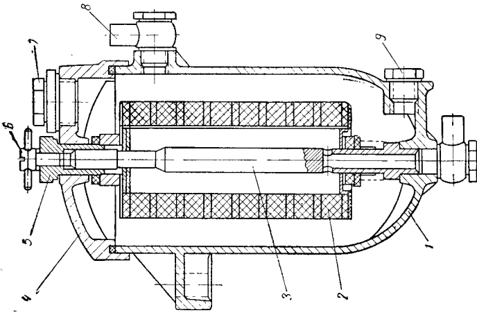
Рис. 20. Топливный фильтр двигателей типа MVD-24:
