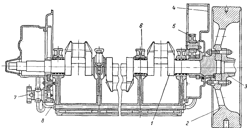
Рис. 8. Коленчатый вал двигателей типа NVD-24 : 1 — коленчатый вал, 2 — маховик, 3 — фланец вала генератора, 4 — корпус регулятора, 5 — шестерня привода кулачкового вала, 6 — верхняя крышка рамового подшипника, 7 — масляный насос, 8 — всасывающая труба масляного насоса.
