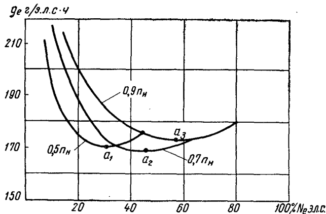
Рис. 56. Нагрузочные характеристики двигателя при n = \text{const} . a_1, a_2, a_3 — точки, которым соответствует наименьший удельный расход топлива.
