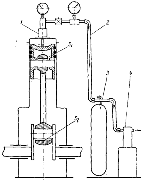
Рис. 101. Схема включения прибора: 1 — прибор, 2 — шланг, 3 — ресивер, 4 — компрессор.
