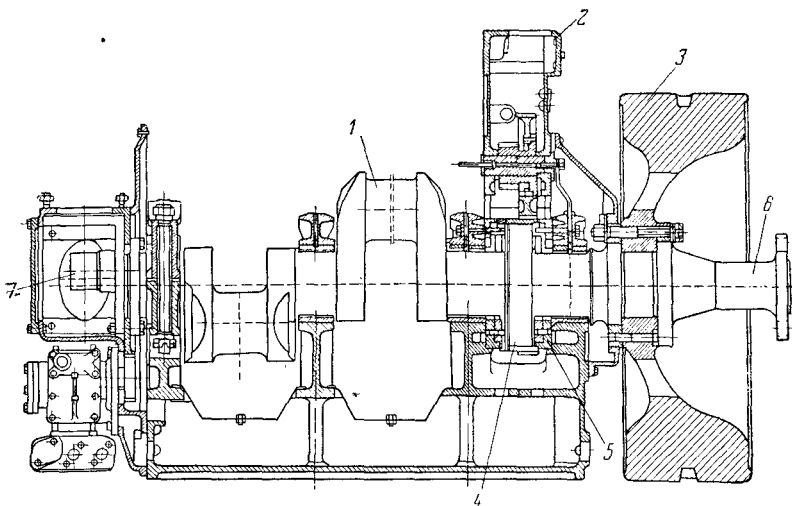
Рис. 7. Коленчатый вал двигателей типа NVD-48 и NVD-36 :
