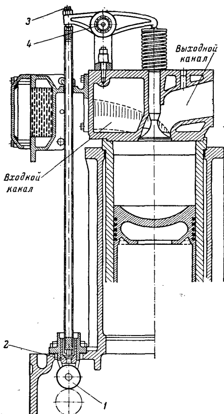
Рис. 13. Привод клапанов:
