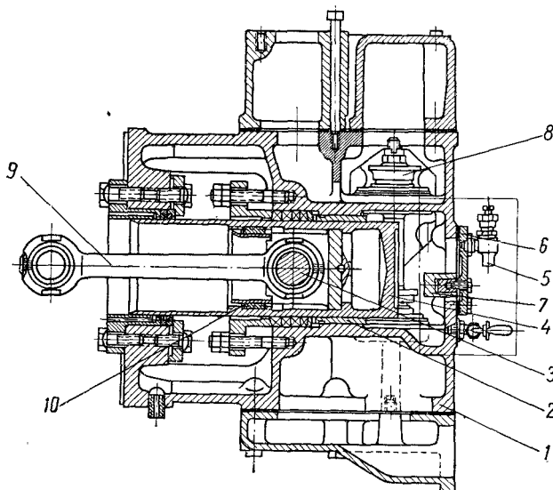
Рис. 52. Охлаждающий насос двигателей типа NVD-48 и NVD-36 :
