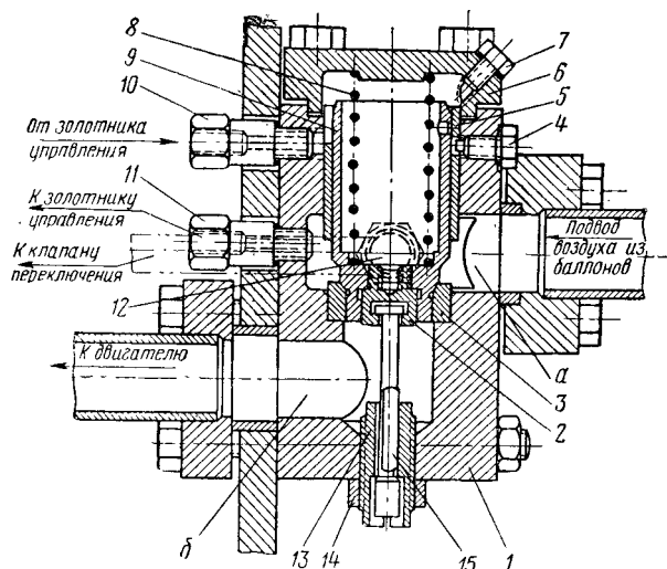
Рис. 34. Главный пусковой клапан двигателей типа NVD-48 и NVD-36:
