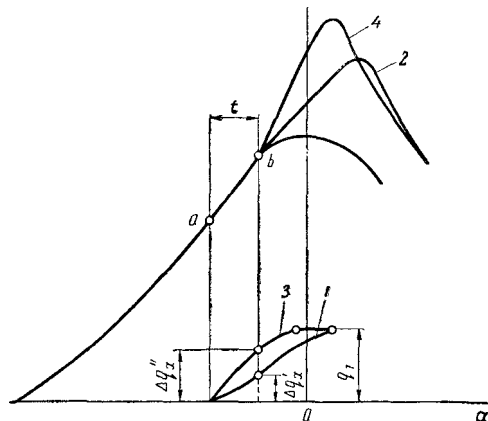
Рис. 119. Влияние закона подачи топлива на площадь индикаторной диаграммы:
