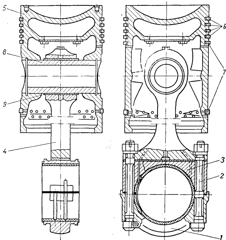
Рис. 9. Шатун (в сборе с поршнем) двигателей типа NVD-48 : 1 — нижняя крышка, 2 — шатунный болт, 3 — верхняя крышка, 4 — стержень шатуна, 5 — поршень, 6 — компрессионные кольца, 7 — масляные кольца, 8 — поршневой палец, 9 — втулка верхней головки шатуна.
