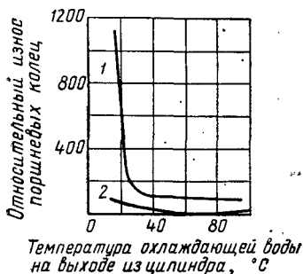
Рис. 66. Влияние температуры охлаждающей воды на износ поршневых колец при различном содержании серы в топливе:
