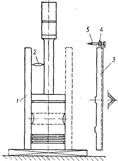
Рис. 98. Проверка перпендикулярности осей шатуна и поршневого пальца:
