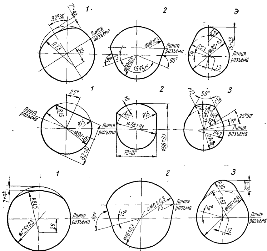
Рис. 105. Профили кулаков:
