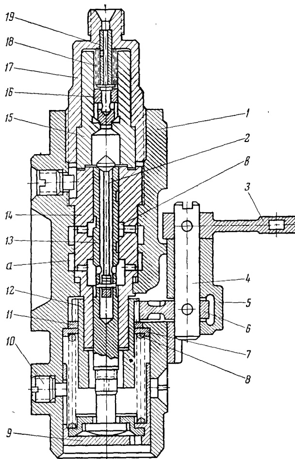
Рис. 22. Топливный насос двигателей типа NVD-24:
