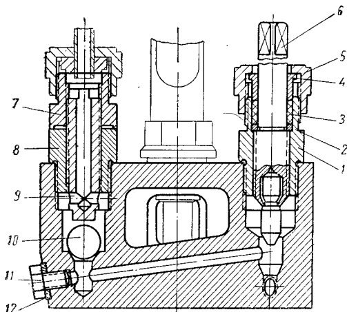
Рис. 40. Газоотборный клапан двигателей типа NVD-24 :
