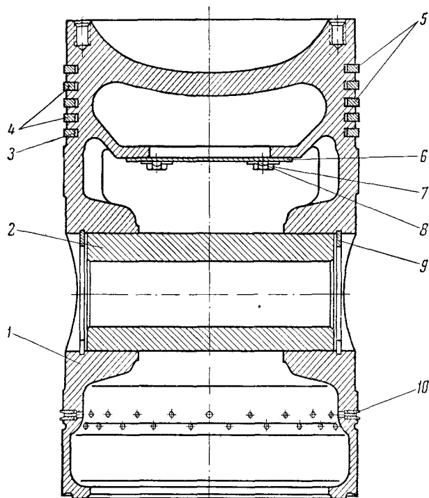
Рис. 12. Поршень (в сборе) двигателей типа NVD-48 : 1 — поршень, 2 — палец поршня, 3 — верхнее маслоъемное кольцо, 4 — компрессионные кольца с правым замком, 5 — компрессионные кольца с левым замком, 6 — крышка, 7 — болт, 8 — стопорная шайба, 9 — стопорное пружинное кольцо, 10 — нижнее маслоъемное кольцо.
