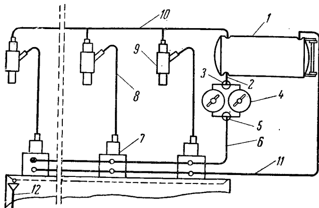
Рис. 18. Схема трубопроводов топливной системы: 1 — расходная топливная цистерна, 2 — топливный трубопровод, 3, 5 — трехходовой кран, 4 — топливный фильтр, 6 — трубопровод, подводящий топливо, 7 — топливный насос высокого давления, 8 — нагнетательный трубопровод, 9 — форсунка, 10, 11, 12 — сливной трубопровод.
