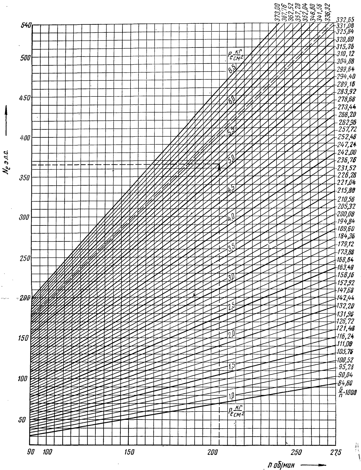
Рис. 115. Номограмма для определения нагрузки на двигатель 8NVD-48 по параметру \frac{G}{n} \cdot 1000 .
