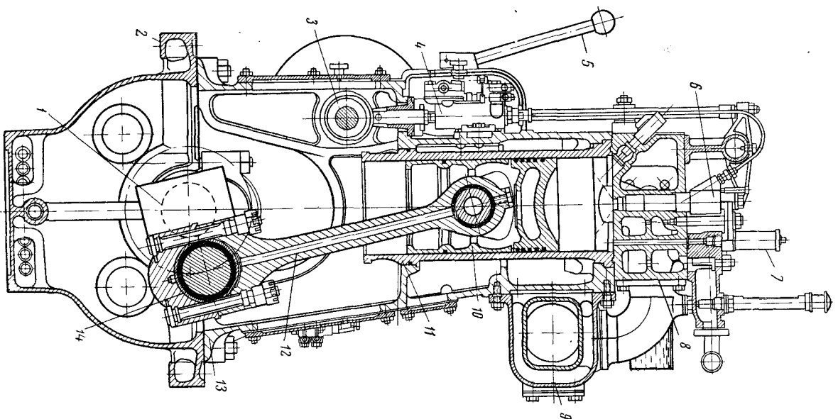
Рис. 3а. Поперечный разрез двигателя типа NVD-24:
