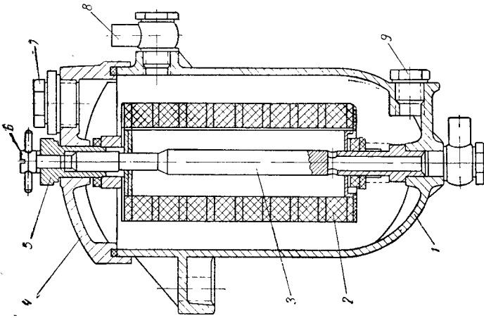
Рис. 20. Топливный фильтр двигателей типа MVD-24:
