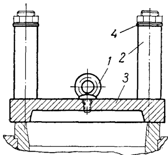
Рис. 92. Приспособление для обжатия втулок цилиндра:
