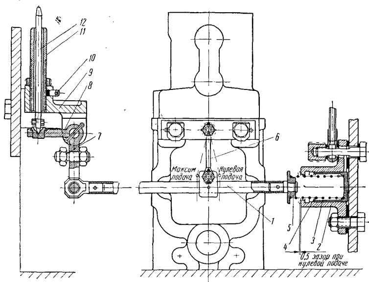
Рис. 30. Привод регулировочной тяги топливных насосов двигателей типа NVD-36:
