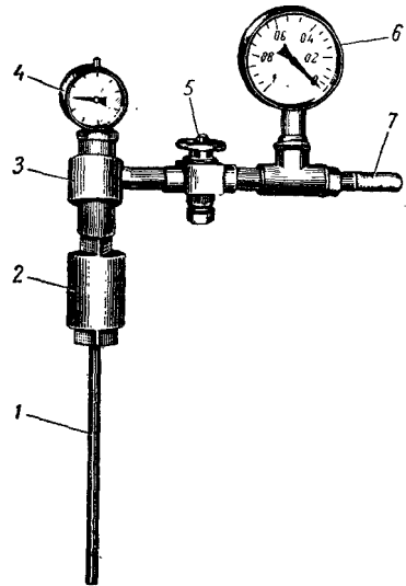
Рис. 102. Прибор для определения зазоров в мотылевом и головном подшипниках:
