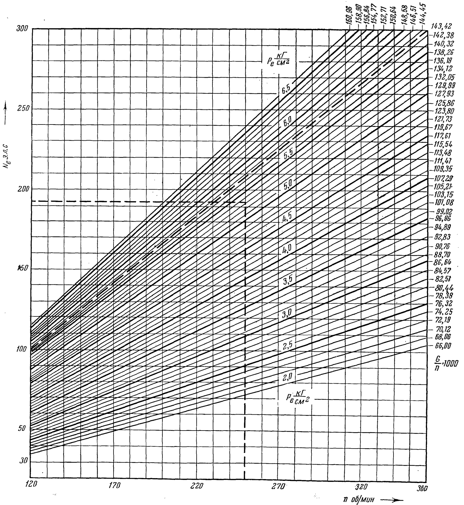
Рис. 117. Номограмма для определения нагрузки на двигатель 8NVD-36 по параметру \frac{G}{n} \cdot 1000 .
