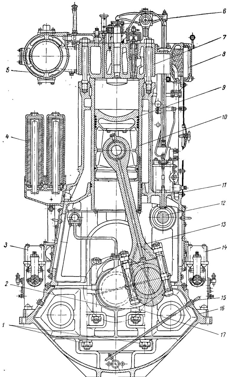
Рис. 1а. Поперечный разрез двигателя типа NVD-48:
