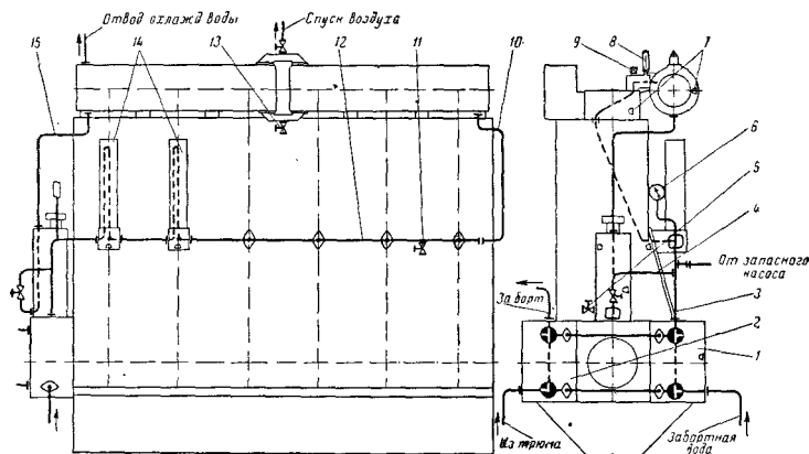
Рис. 51. Система охлаждения забортной водой двигателей типа NVD-48 и NVD-36 :
