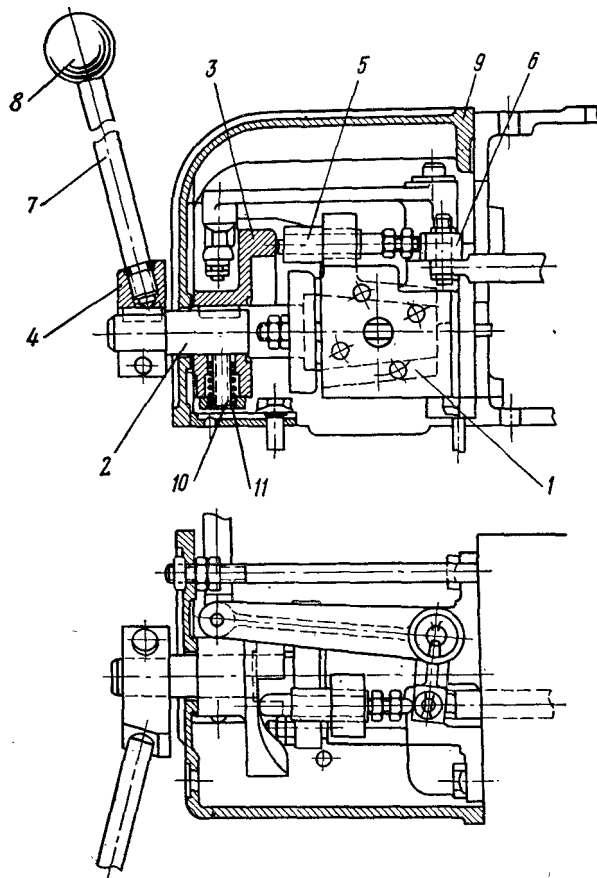
Рис. 43. Пост управления двигателями типа NVD-24 :
