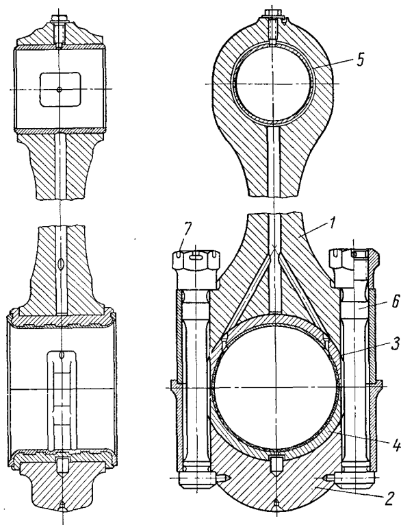
Рис. 10. Шатун (в сборе) двигателей типа NVD-36 :
