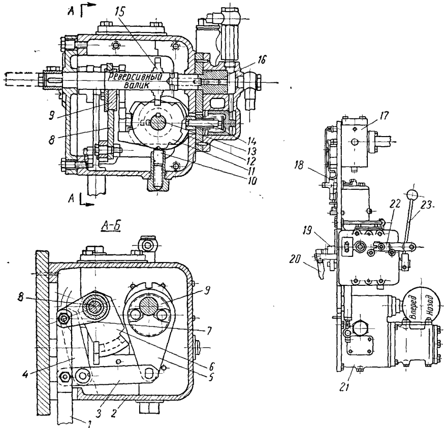
Рис. 41. Пост управления двигателями типа NVD-48:
