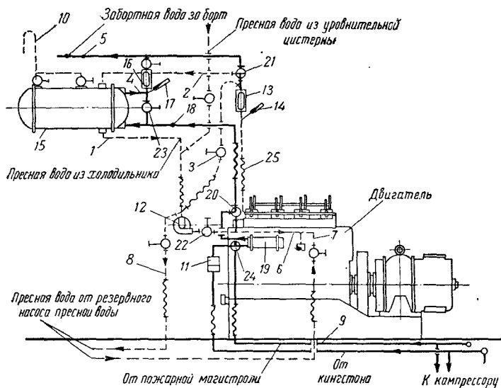
Рис. 54. Система охлаждения двигателей типа NVD-24 пресной водой:
