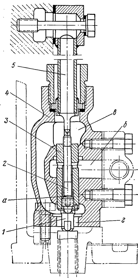
Рис. 38. Распределительный воздушный золотник двигателей типа NVD-24 :
