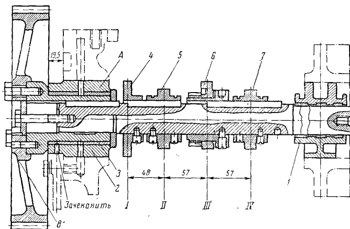
Рис. 17. Распределительный вал двигателей типа NVD-24 :
