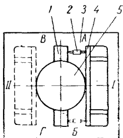
Рис. 95. Проверка пересечения осей пальца и поршня с помощью угольника и микрометрического штихмасса:
