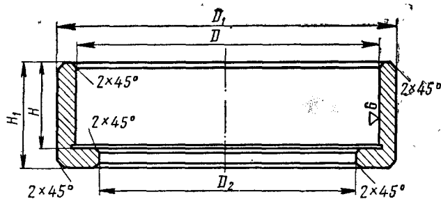
Рис. 2. Калибр (фальшштулка).
