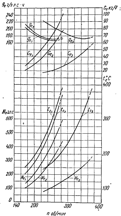
Рис. 114. Результаты испытаний двигателей на контрольном ходу судна.
