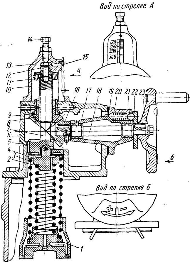
Рис. 28. Пружинные весы регулятора числа оборотов двигателей типа NVD-36 :
