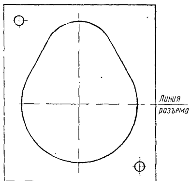
Рис. 104. Типовая форма шаблона кулачной шайбы.
