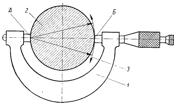
Рис. 83. Пример обмера шейки коленчатого вала микрометрической скобой:
