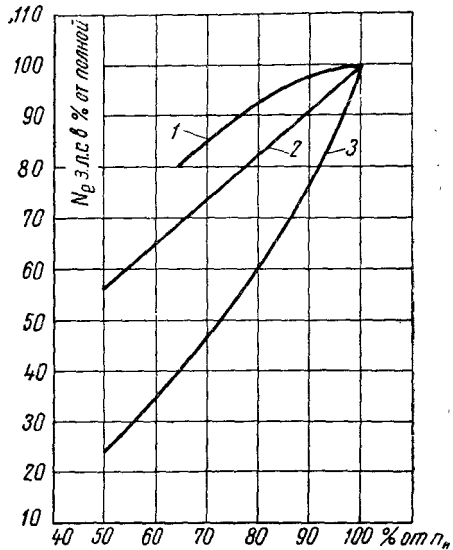
Рис. 55. Скоростные характеристики двигателя:
