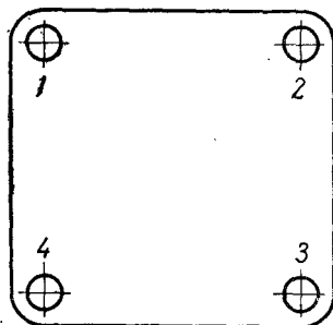
Рис. 82. Условная нумерация шпилек крепления цилиндрических крышек двигателей типа NVD-36 и NVD-24 .
