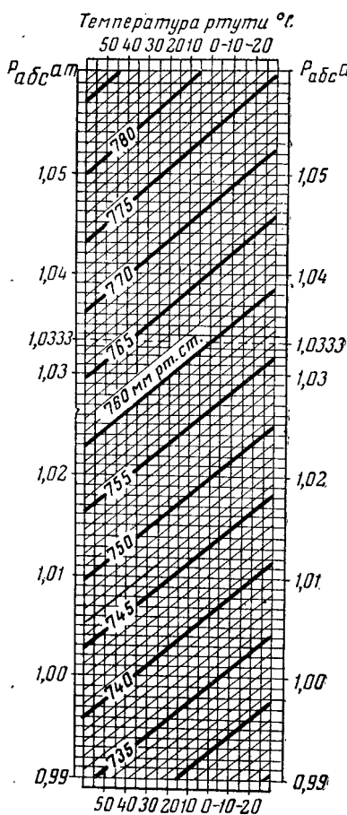
Рис. 65. Номограмма барометрического давления.
