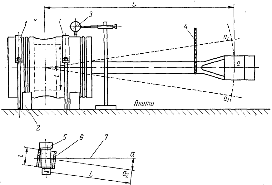
Рис. 100. Определение зазора в головном подшипнике при снятом поршне: 1 — скоба для крепления, 2 — призмы, 3 — индикатор, 4 — струпа, 5 — поршневой палец, 6 — вкладыш головной подшипника, 7 — ось стержня шатуна.
