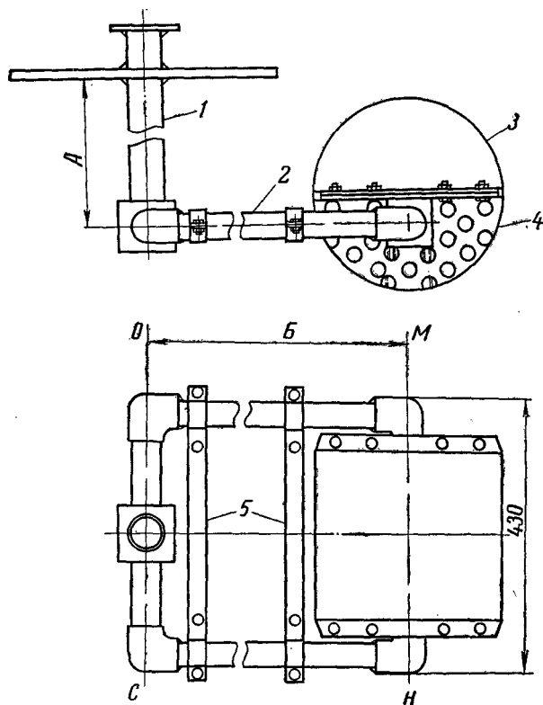
Рис. 120. Поплавковый приемник топлива:
