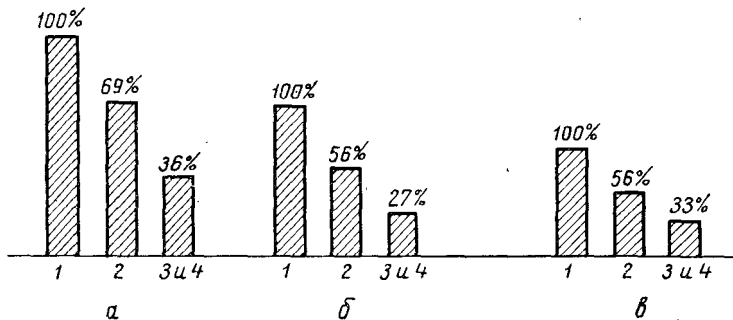
Рис. 78. Соотношение величин износа для двигателя 8NVD-36:
