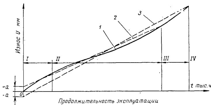
Рис. 79. Динамика износа деталей.
