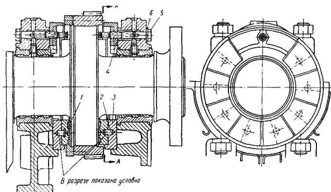
Рис. 4. Упорный подшипник двигателей типа NVD-48 и NVD-36 :
