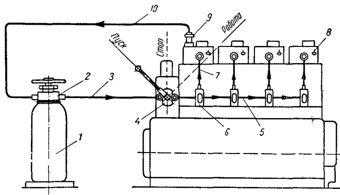
Рис. 33. Схема пусковой системы двигателей типа NVD-24 : 1 — баллон пускового воздуха, 2 — запорный клапан пускового баллона, 3, 7 — трубопроводы, 4 — главный пусковой клапан, 5 — воздушный распределительный коллектор, 6 — распределительные золотники, 8 — пусковые клапаны, 9 — газоотборный клапан, 10 — трубопровод отбора газа.
