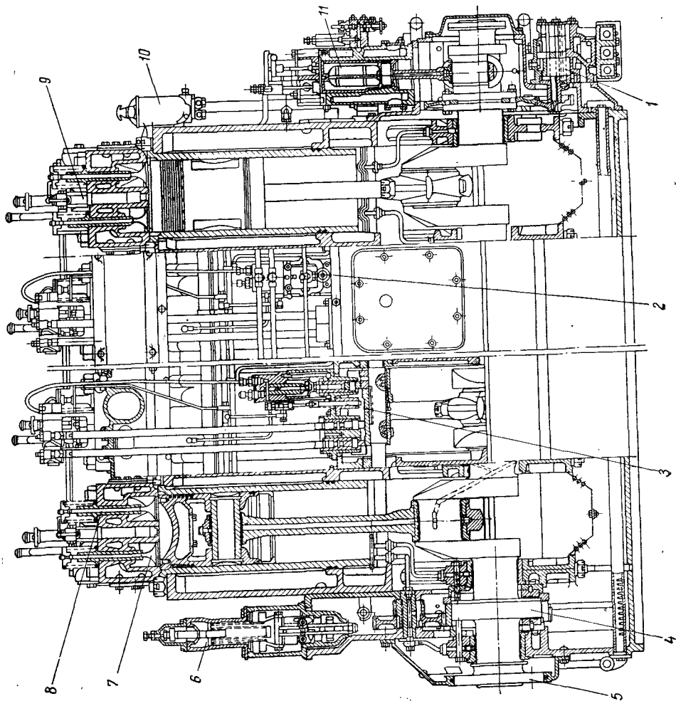
Рис. 2. Продольный разрез двигателя типа VUD-36.
