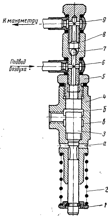
Рис. 36. Пусковой золотник двигателей типа NVD-48 и NVD-36 :
