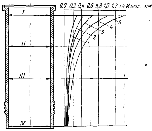
Рис. 70. Износ (по диаметру) втулок рабочих цилиндров двигателя 8NVD-36: 1, 2, 3, 4, 5 — кривые износа втулок соответственно после 2000, 5000, 10000, 15000, 20000 ч работы двигателя.
