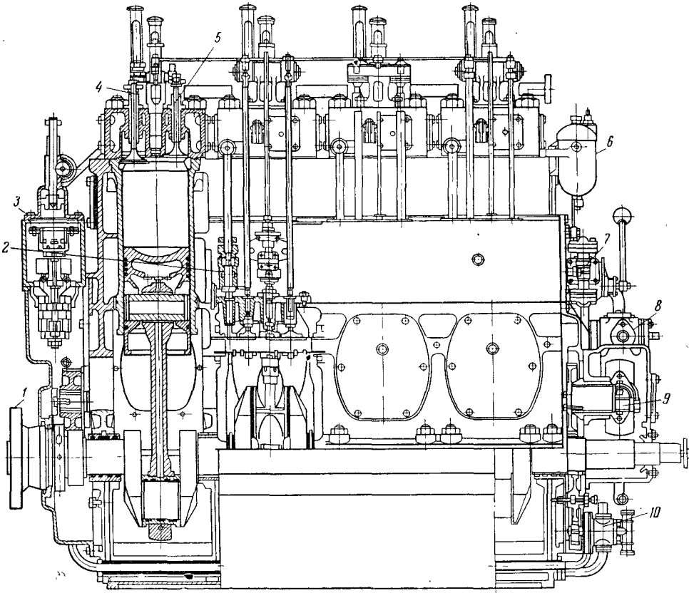
Рис. 3. Продольный разрез двигателя типа NVD-24:
