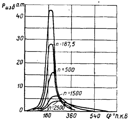
Рис. 77. Влияние числа оборотов двигателя на процесс изменения давления за вторым поршневым кольцом.
