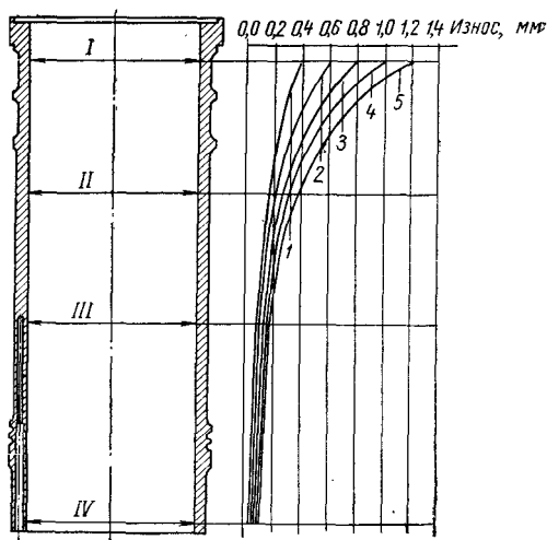
Рис. 69. Износ (по диаметру) втулок рабочих цилиндров двигателя 6NVD-48: 1, 2, 3, 4, 5 — кривые износа втулок соответственно после 2000, 5000, 10000, 15000, 20000 ч работы двигателя.
