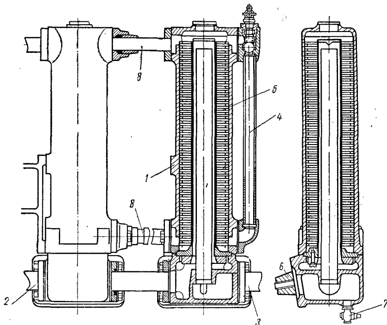
Рис. 49. Маслоохладитель двигателей типа NVD-48 и NVD-36 : 1 — корпус радиатора, 2 — подводящая водяная труба, 3 — отводящая водяная труба, 4 — обходной трубопровод, 5 — набор пластин, 6 — протектор, 7 — спускной кран, 8 — перепускной масляный трубопровод.
