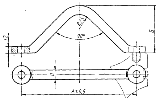
Рис. 85. Скоба для подъема поршня с шатуном.
