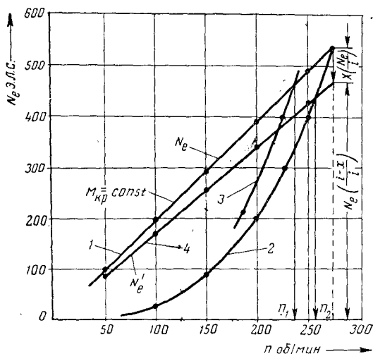
Рис. 57. Скоростные характеристики работы двигателя 8 NVD -48:
