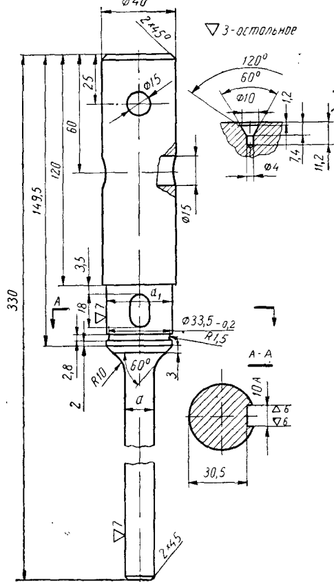
Рис. 108. Шток шарошки.
