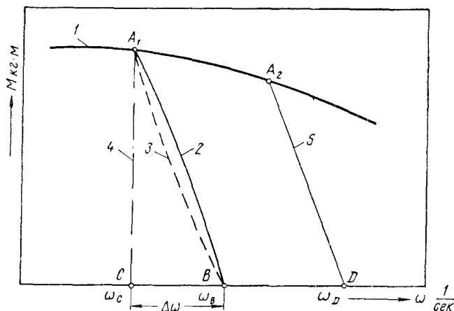
Рис. 62. Характеристики двигателя: 1 — внешняя, 2, 3, 4, 5 — регуляторные статические.
