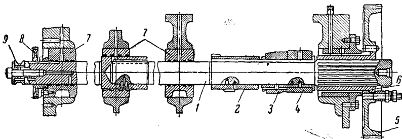
Рис. 15. Распределительный вал двигателей типа NVD-48:
