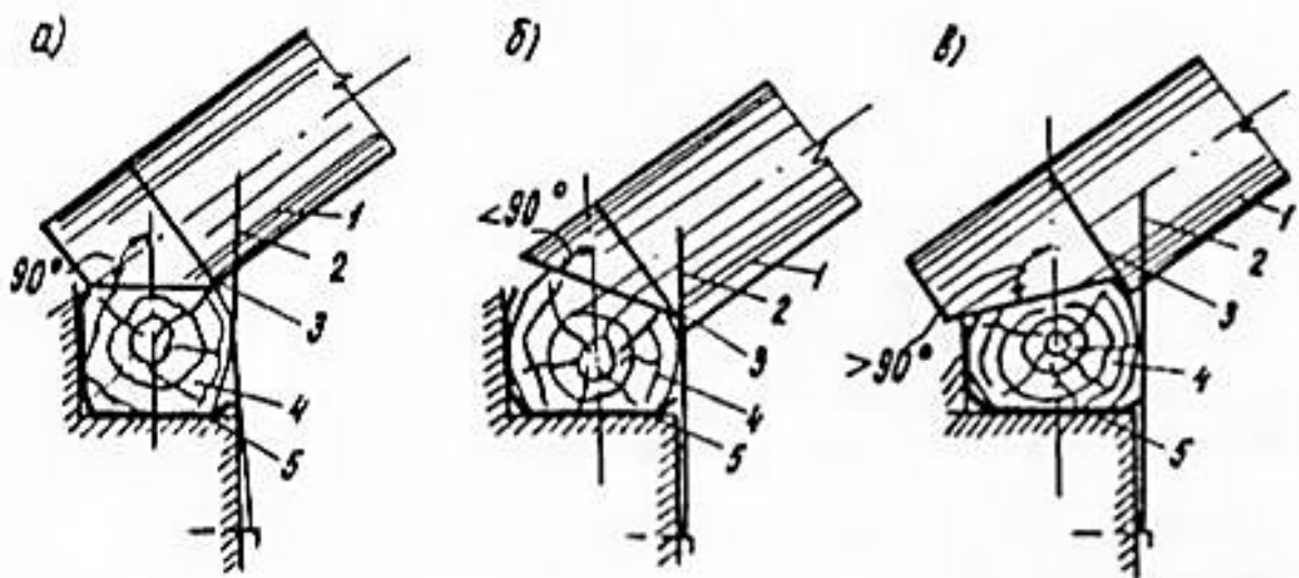
Рис. 38. Правильное (а) и неправильное (б) и (в) выполнение опирания стропильной ноги на мауэрлат: 1 — стропильная нога; 2 — угловая скоба; 3 — скрутка; 4 — мауэрлат; 5 — рулонный гидроизоляционный материал
