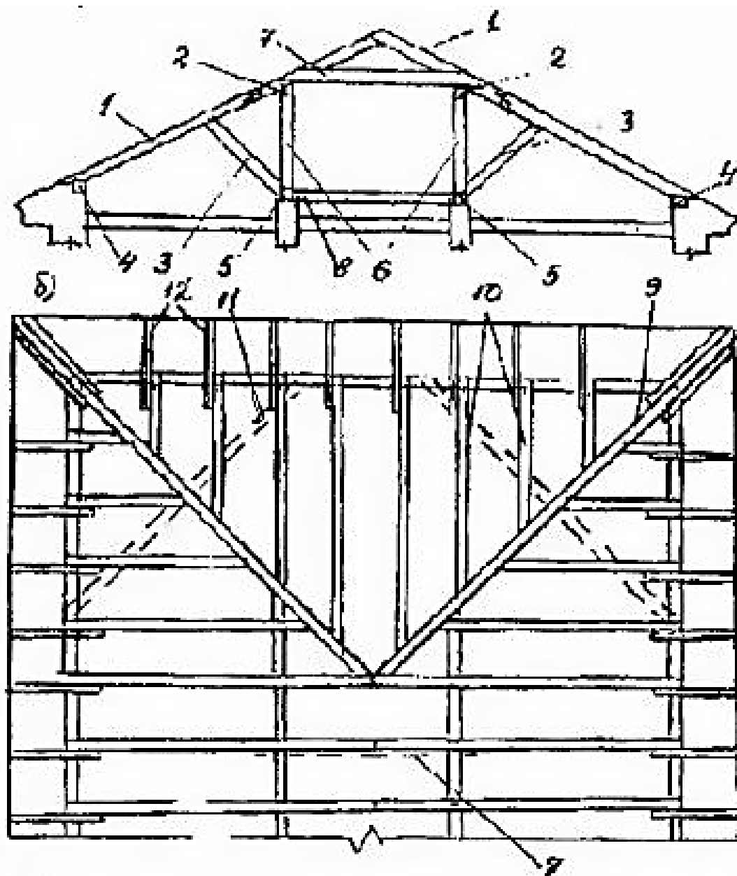
Рис. 3. Схема деревянных наклонных стропил: а — поперечное сечение крыши; б — план стропил; 1 — стропильная нога; 2 — прогон; 3 — подкосы; 4 — мауэрлат; 5 — лежни; 6 — стойки; 7 — ригель; 8 — распорка; 9 — диагональная (накосная) стропильная нога; 10 — нарожки; 11 — шпренгель; 12 — кобылки
