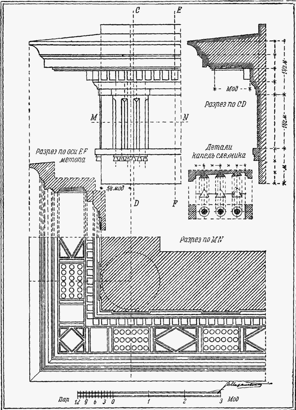
Римско дорический ордер с зубцами — плафон
