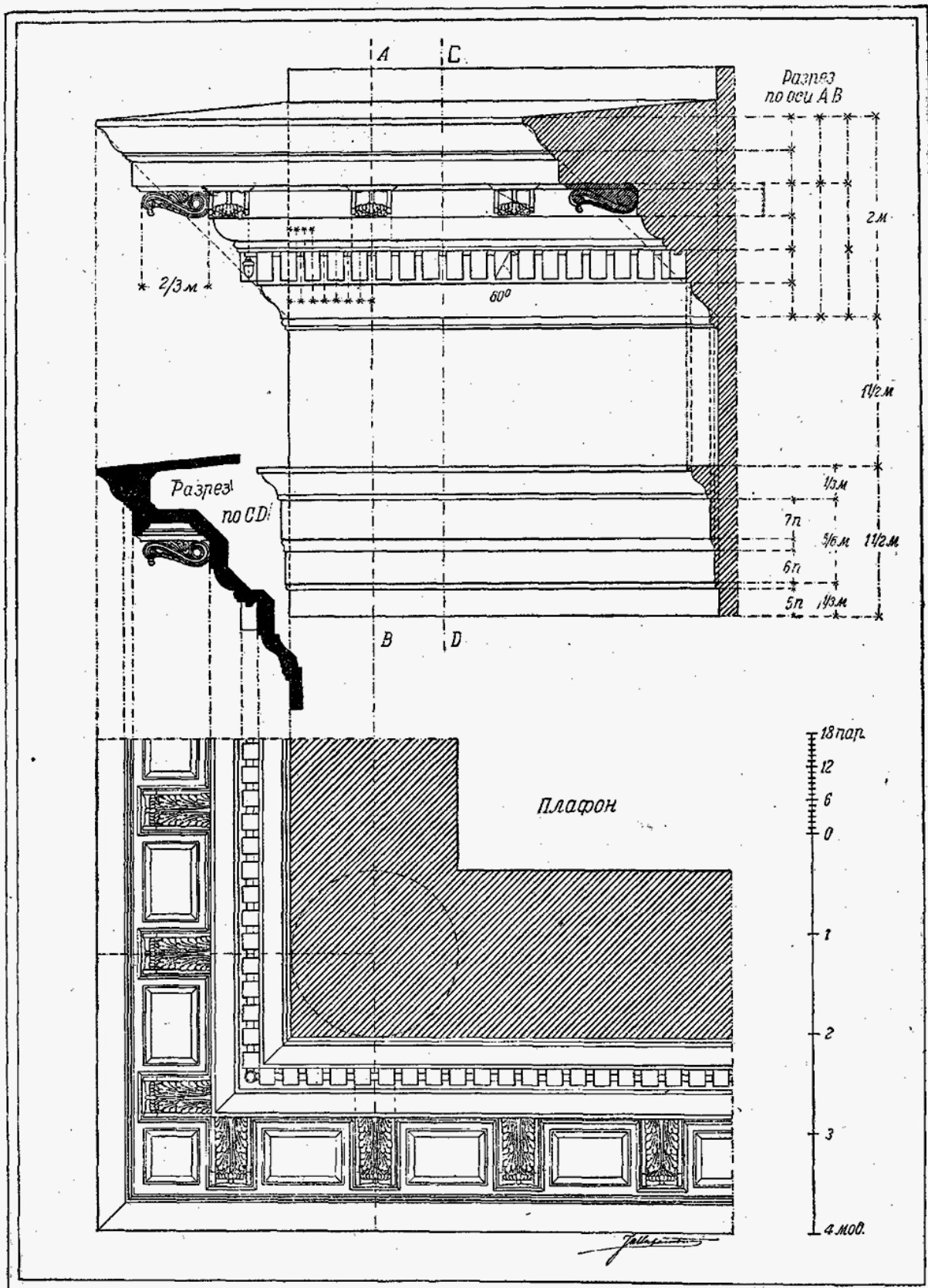
Римско-коринфский ордер — плафон
