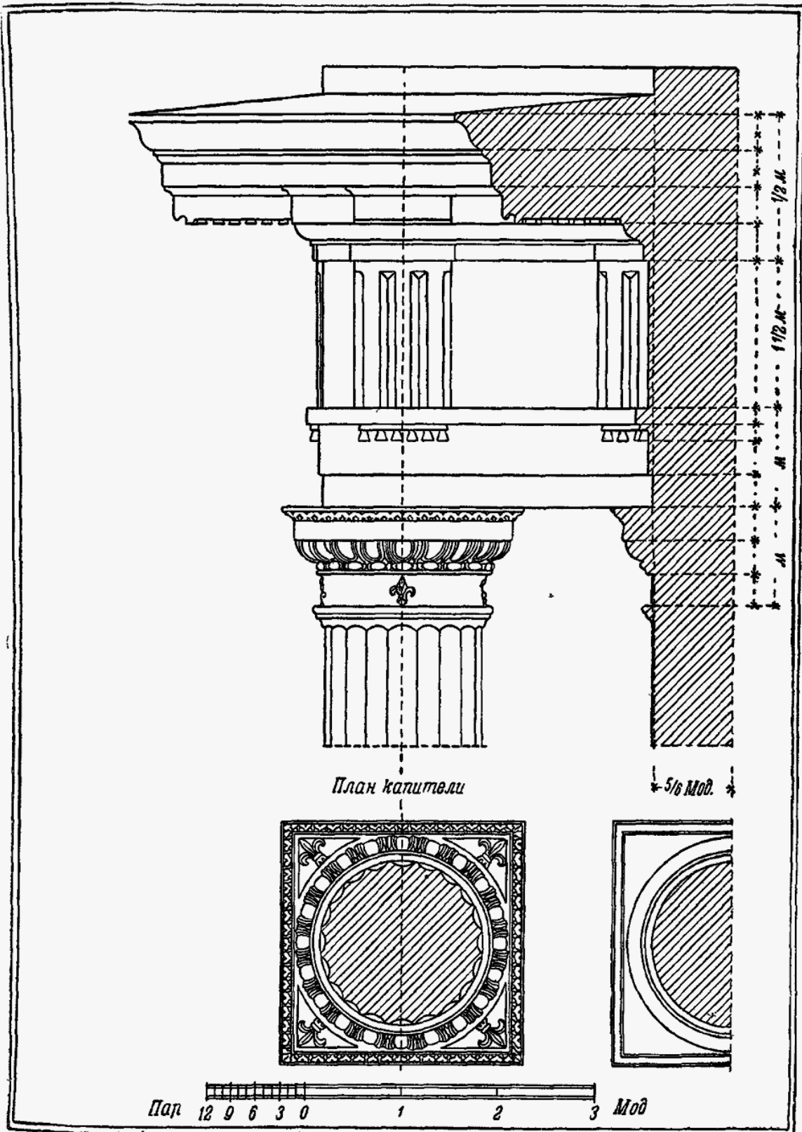
Римско-дорический ордер с модульонами — антаблемент и капитель
