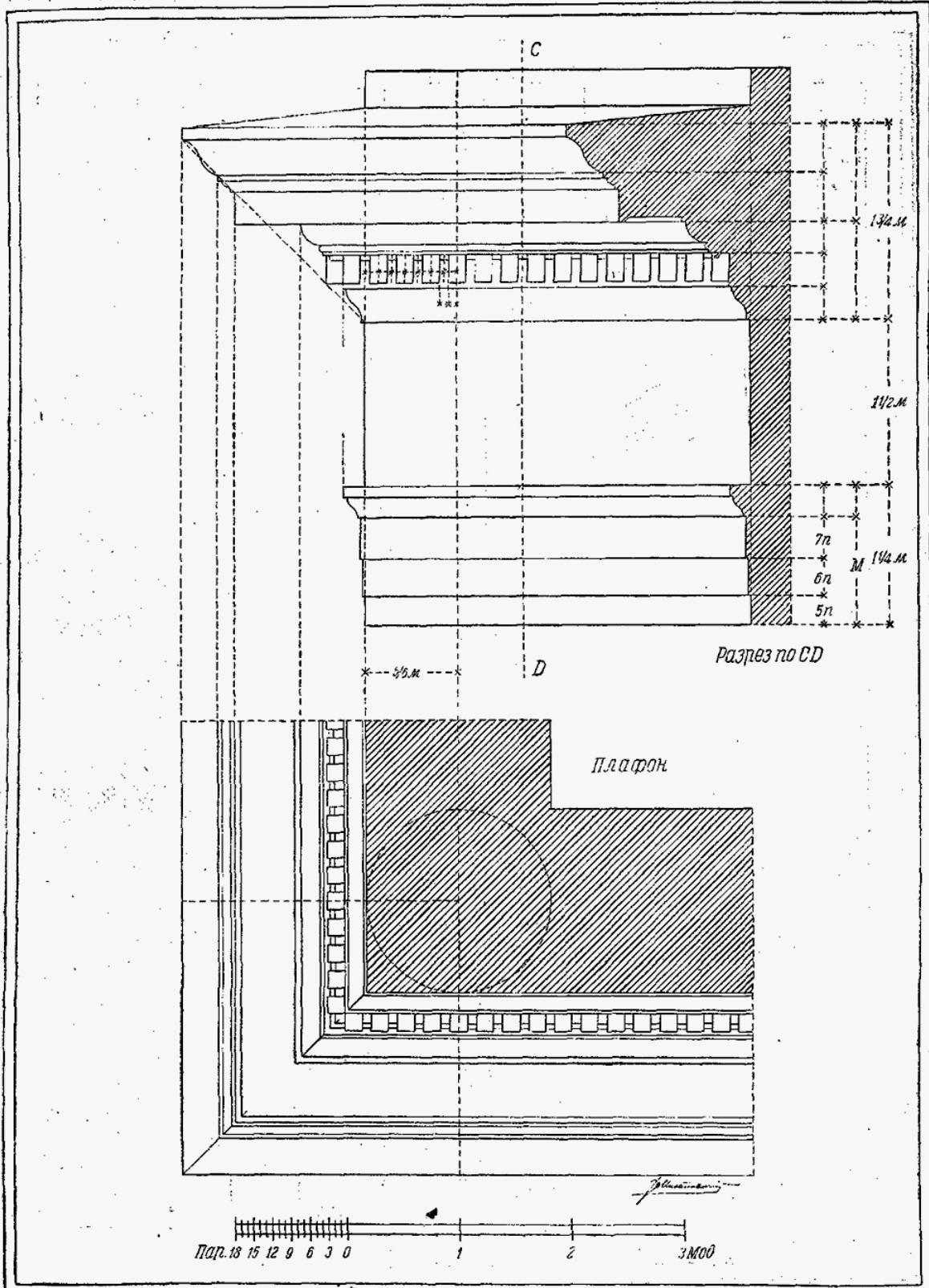
Римско-ионический ордер — плафон
