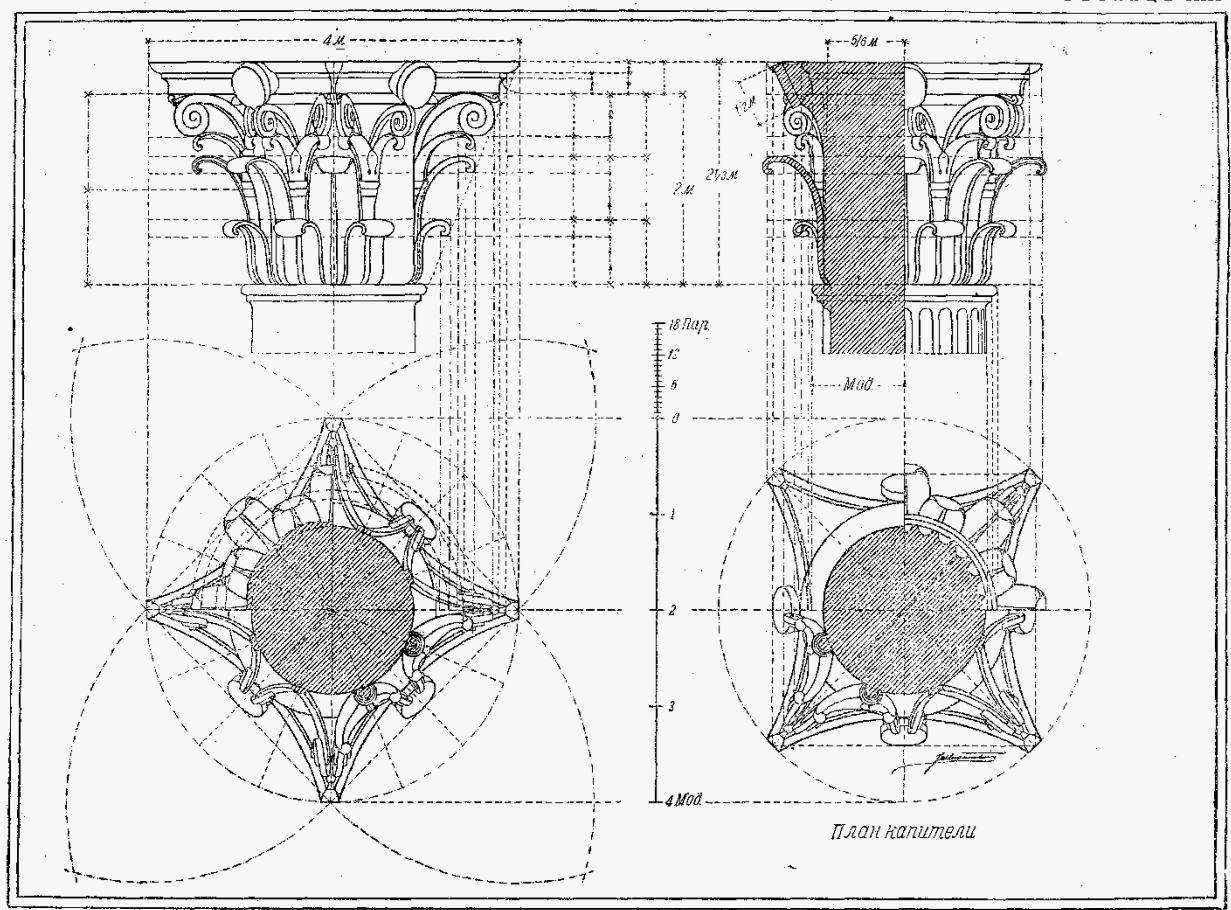
Построение римско-коринфской капители
