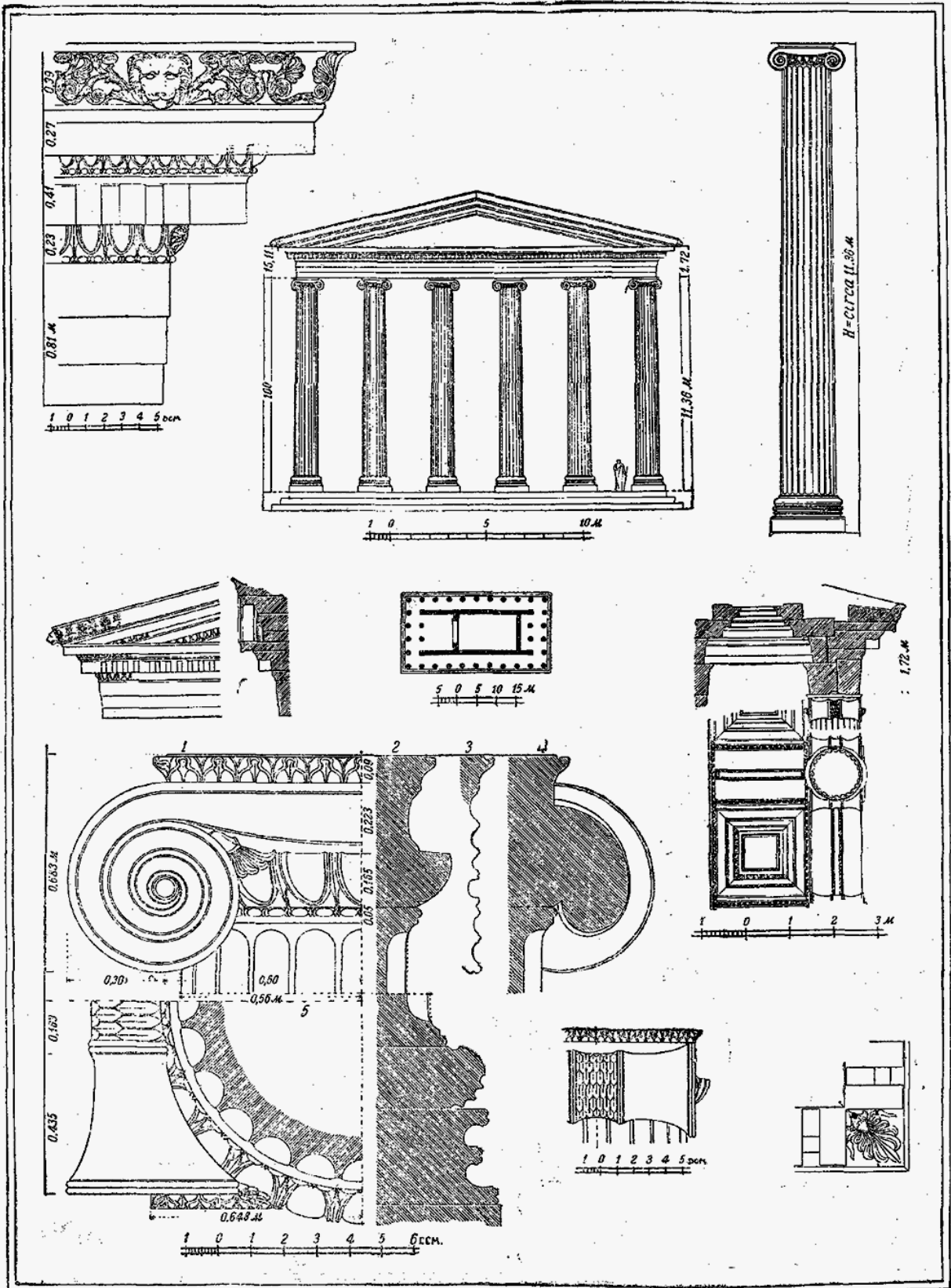
Греко-ионический ордер. (Храм в Приене, Малая Азия)
