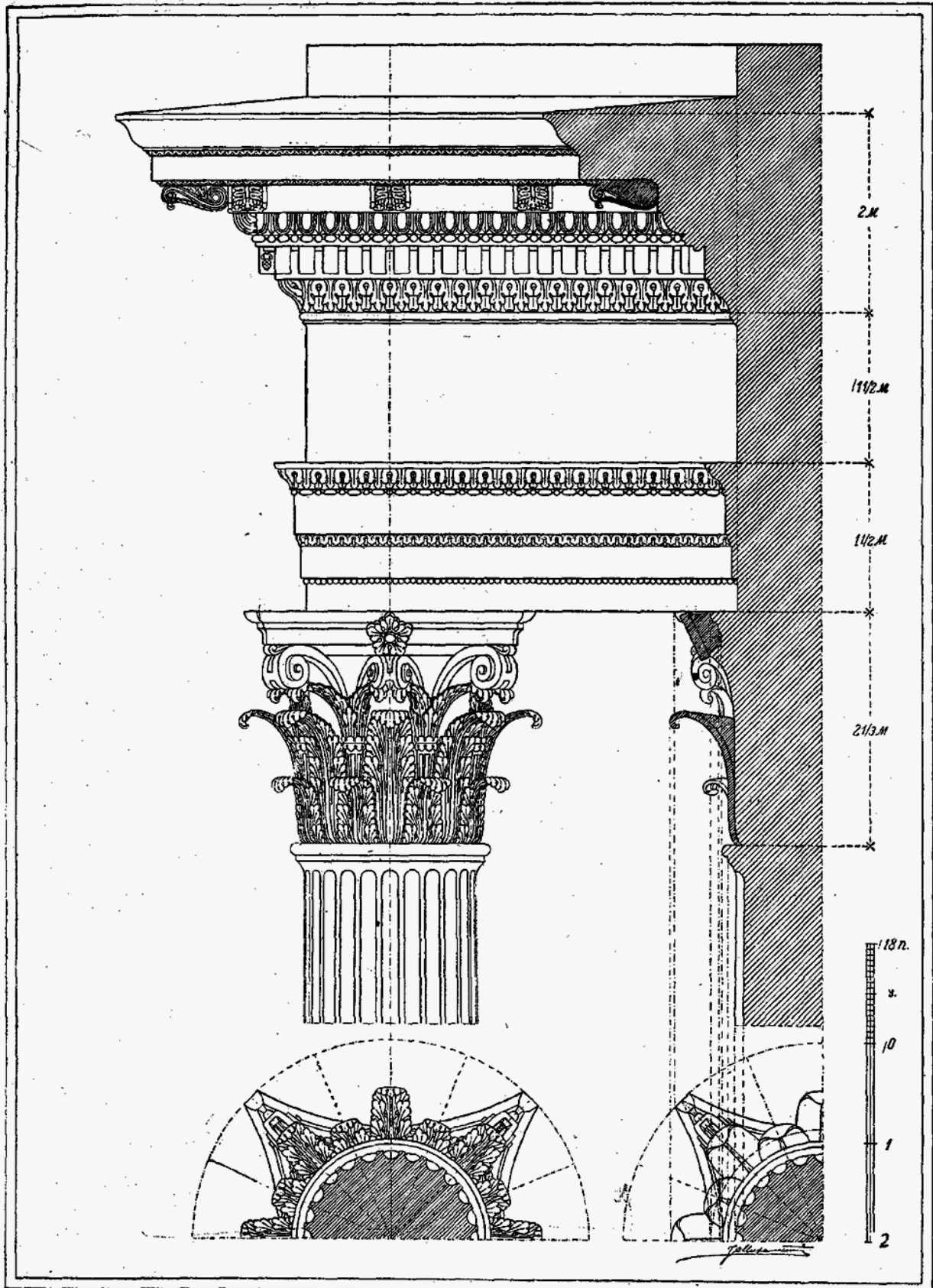
Римско-коринфский ордер — антаблемент и капитель
