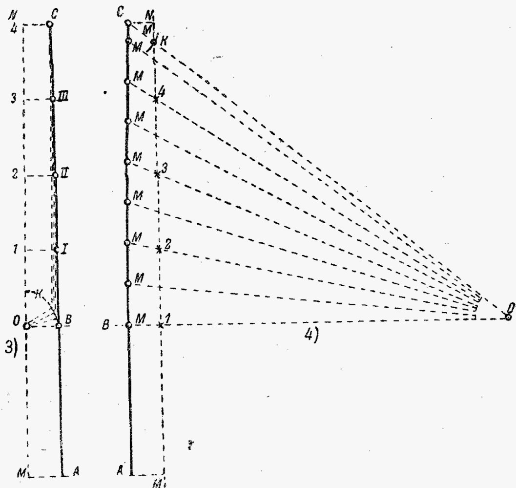
Рис. 3 и 4. Построение утонения колонны
