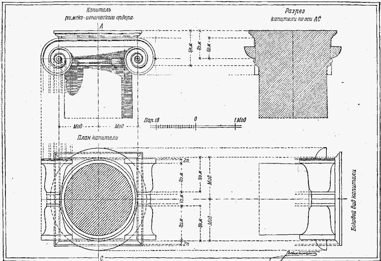
Римско-ионический ордер — капитель
