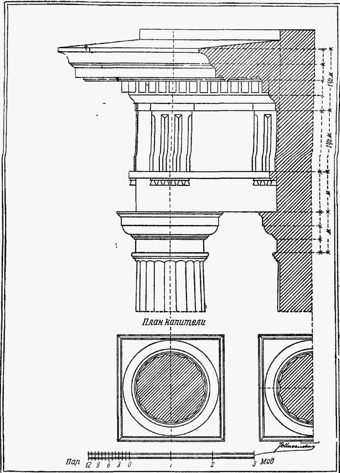
Римско-дорический ордер с зубцами — антаблемент и капитель
