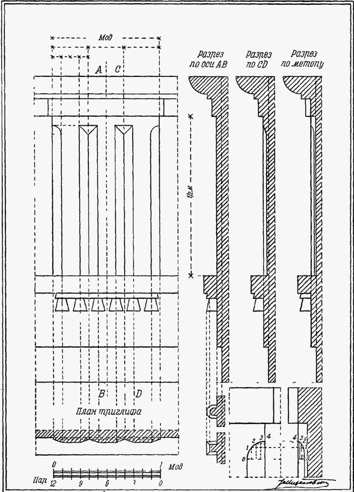
Римско-дорический ордер — детали триглифа
