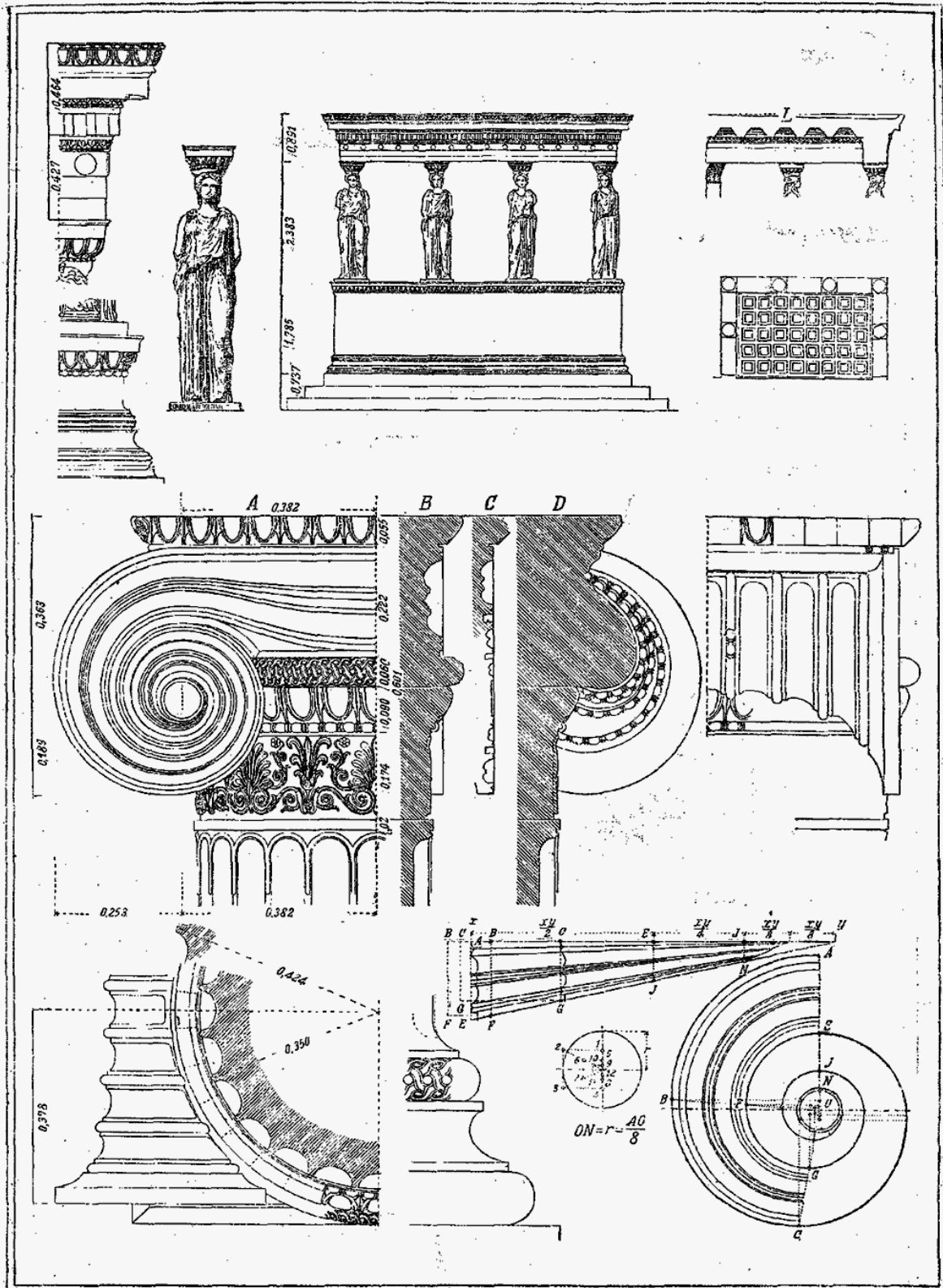
Греко-ионический ордер (Эрехтейон)
