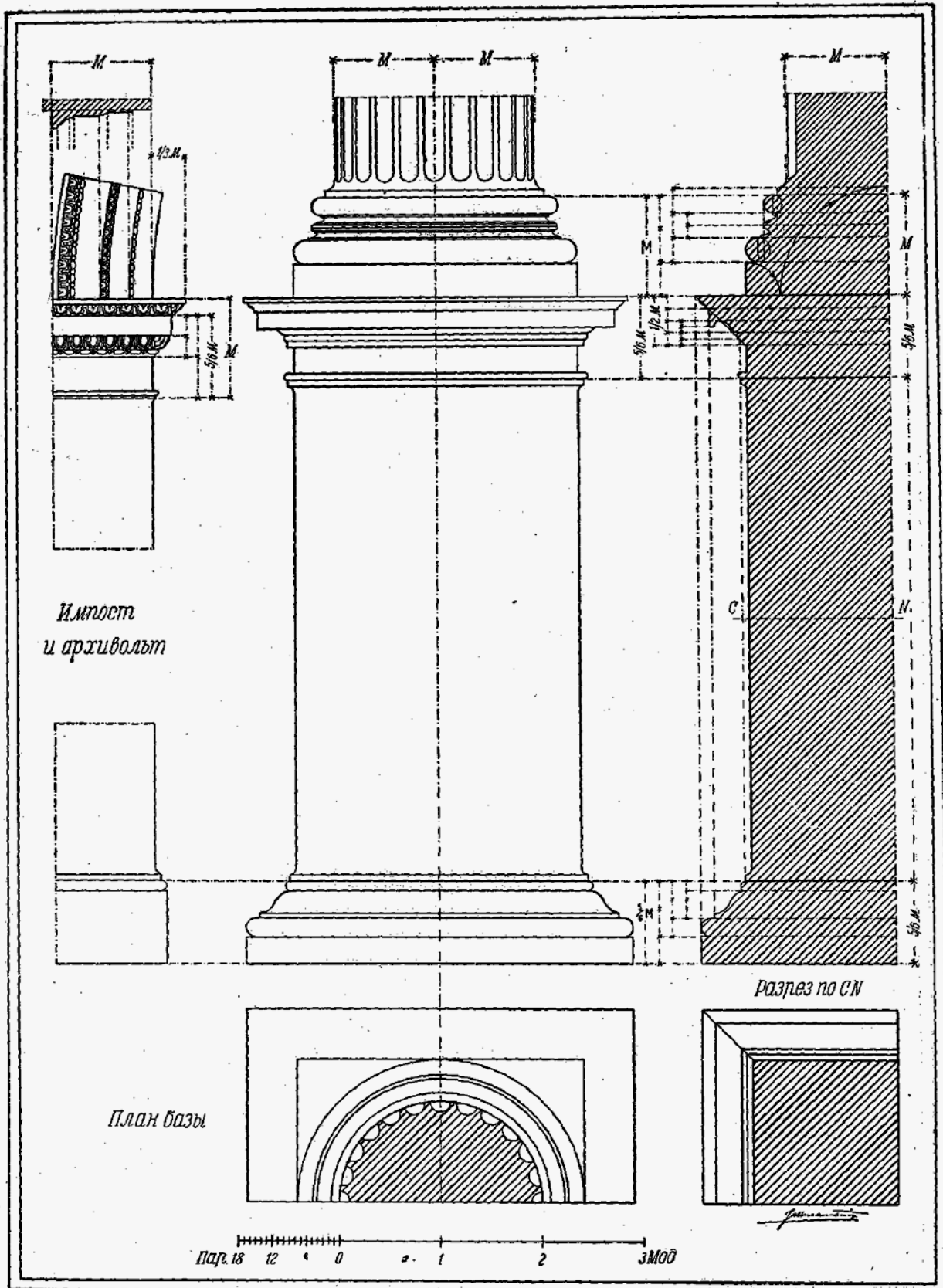
Римско-коринфский ордер — база и постелит
