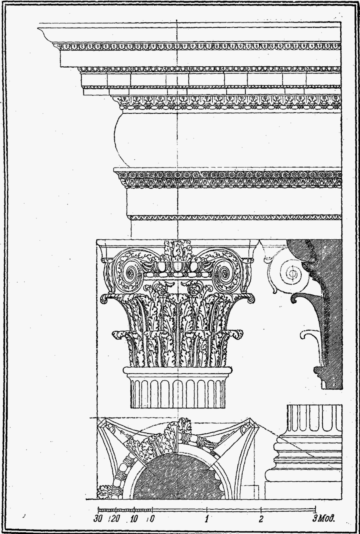
Сложный ордер (по Палладио)
