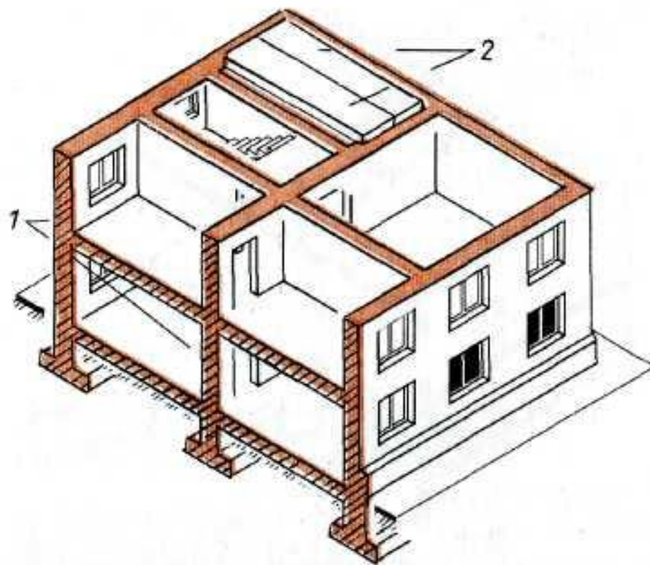
33. ЗДАНИЕ БЕСКАРКАСНОГО ТИПА 1 – несущие стены; 2 – междуэтажные перекрытия
