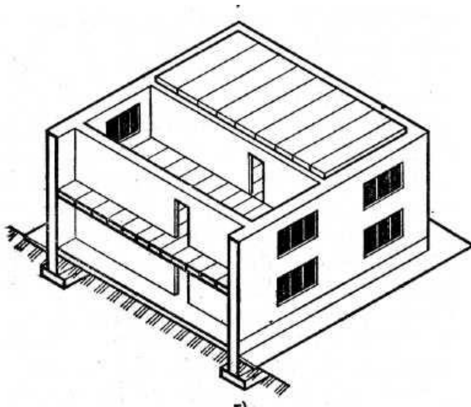
С поперечными несущими стенами
