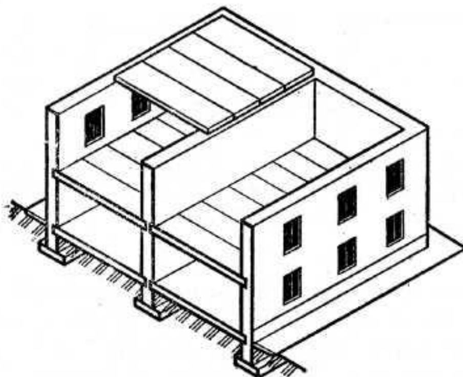
С продольными несущими стенами
