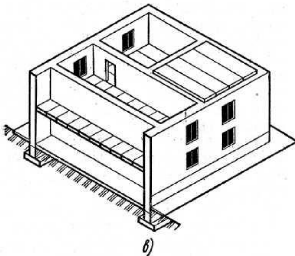
Перекрестно-стеновая система
