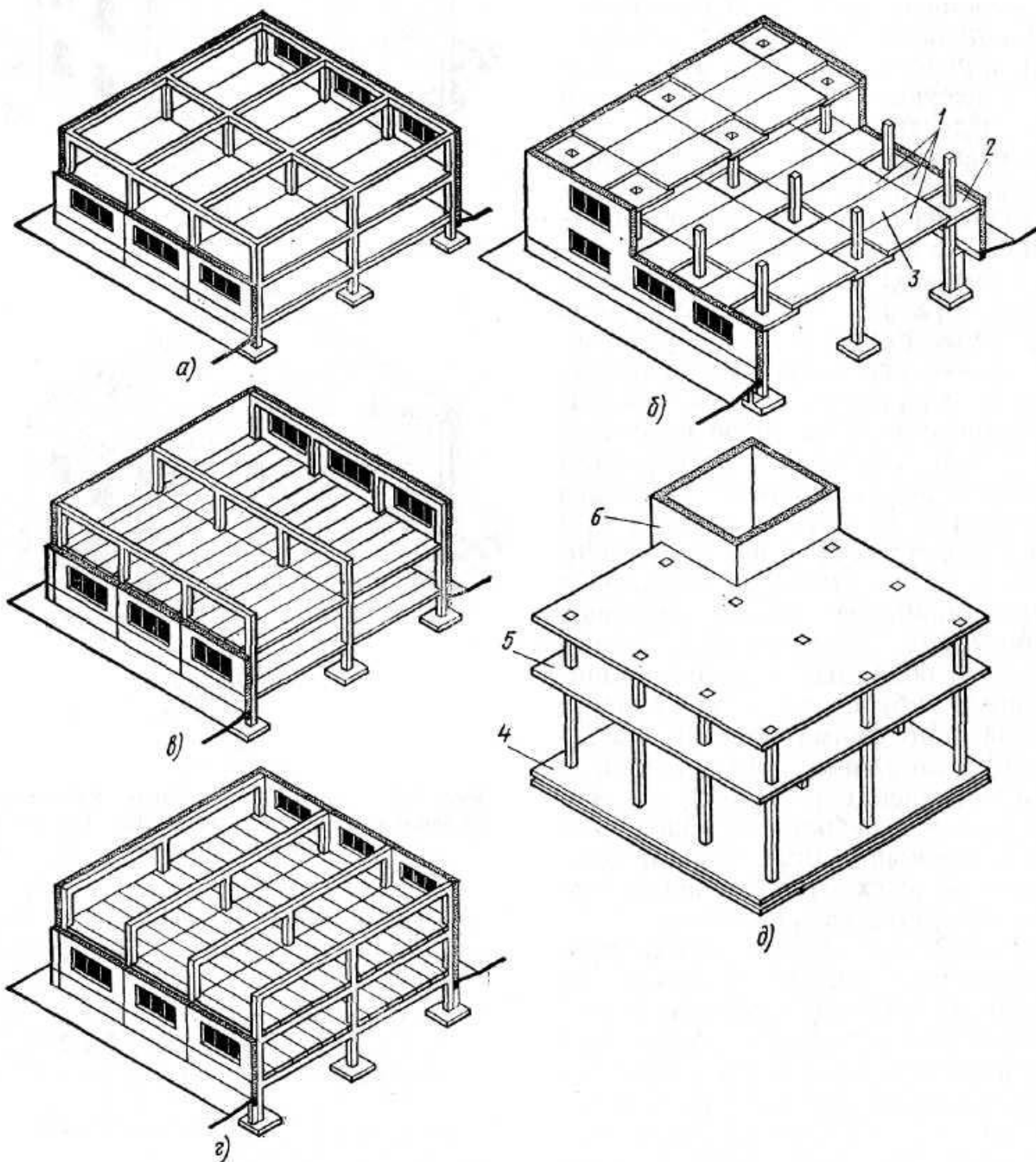
Рис. 15. Конструктивные схемы каркасных зданий:
