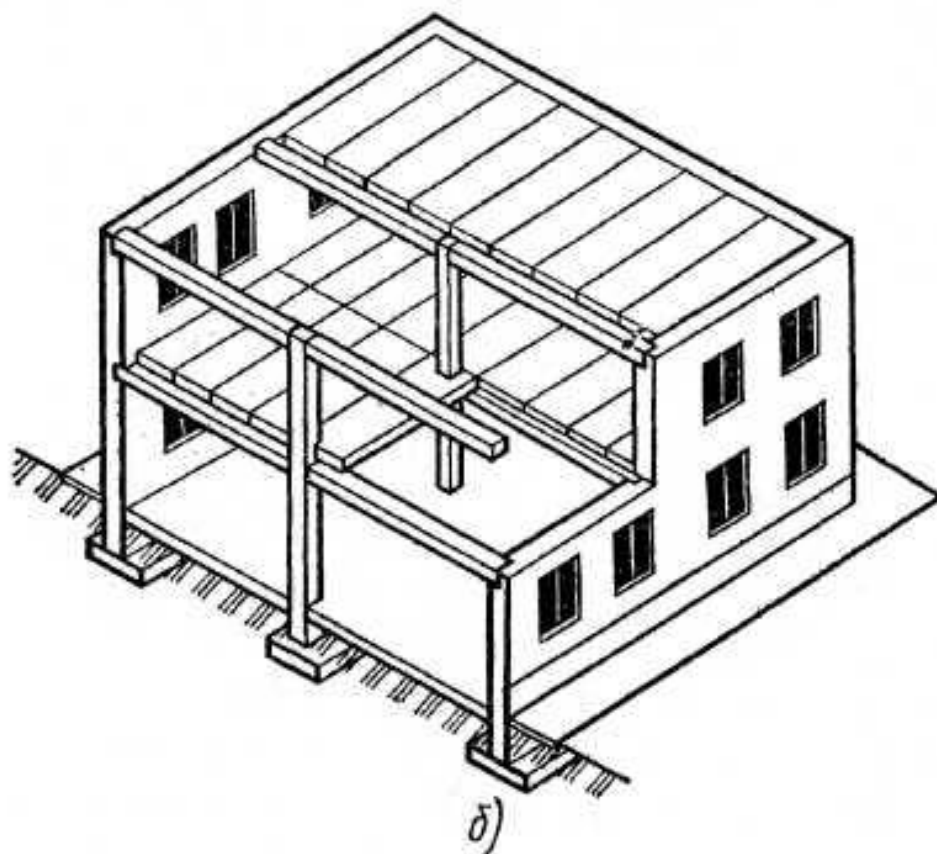
Рис. 13. Здания с неполным каркасом с продольным (а) и поперечным (б) расположением ригелей
