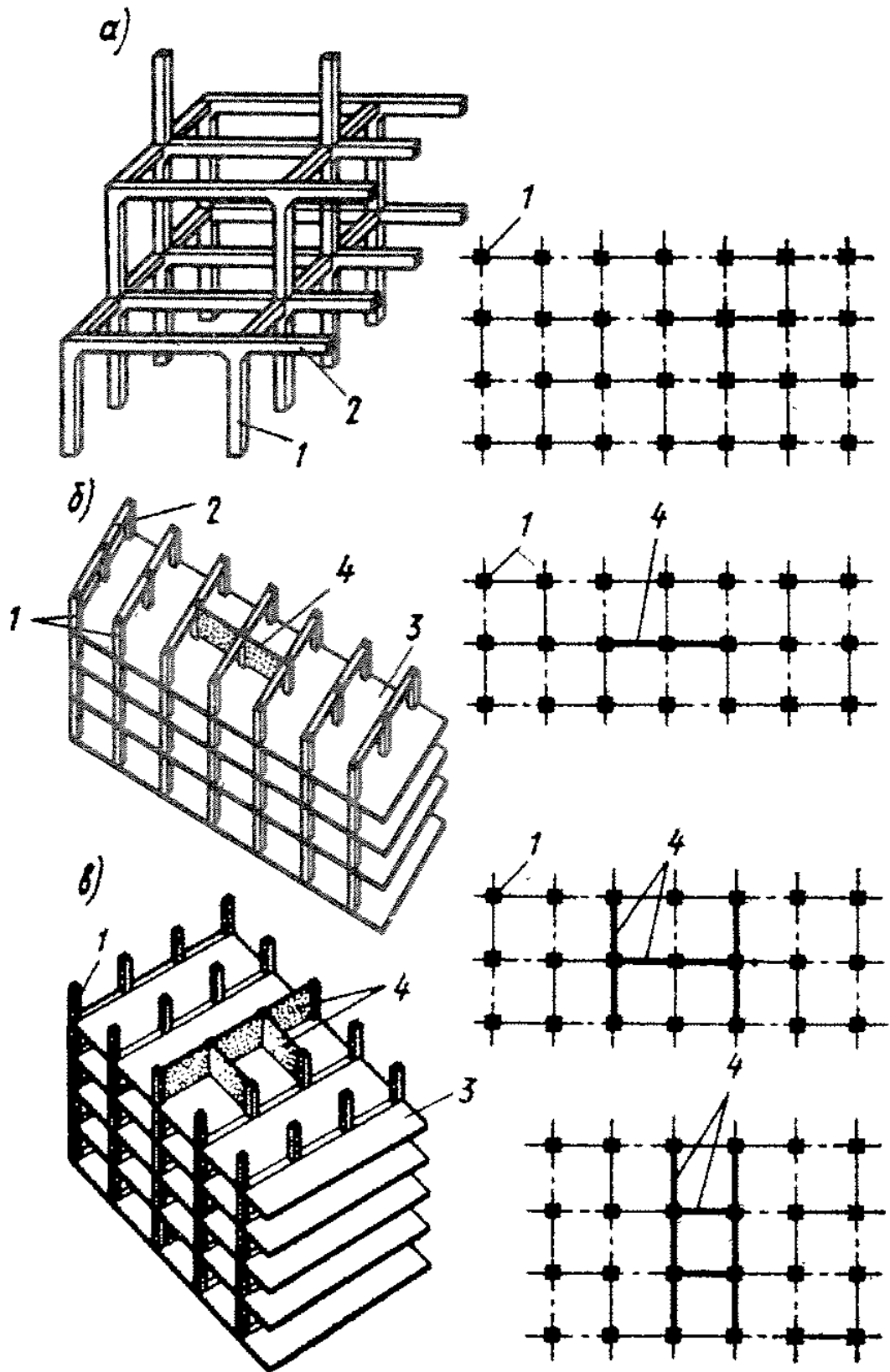
Рис. II.9. Конструктивные схемы каркасов: а — рамная; б — рамно-связевая; в — связевая; 1 — колонна; 2 — ригель; 3 — жесткий диск перекрытия; 4 — диафрагма жесткости
