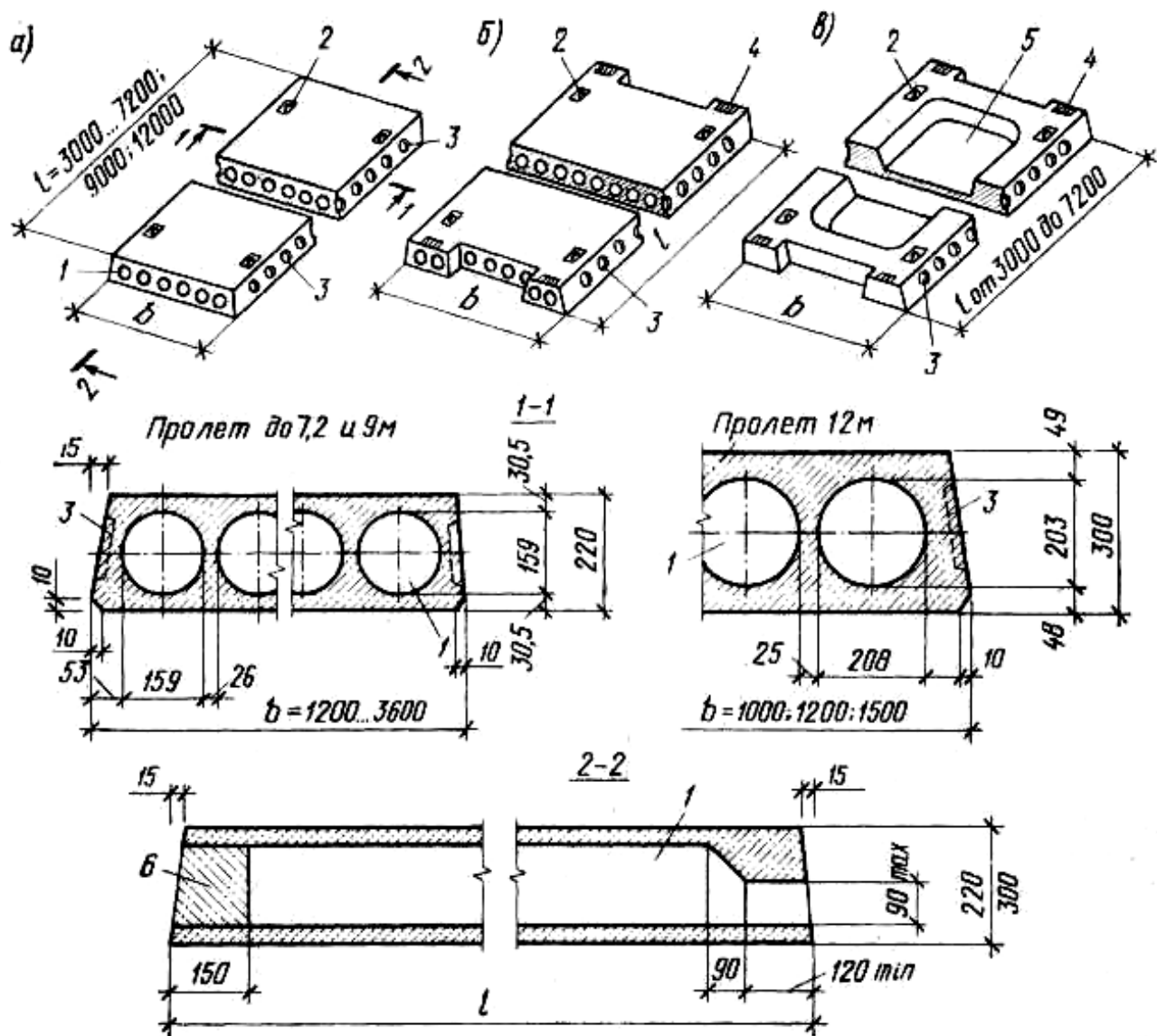
Плиты железобетонные многопустотные для перекрытий жилых и общественных зданий: a — рядовая плита; б — плита-распорка внутренняя; в — санитарно-техническая «корытная» плита-распорка; / — пустоты плиты; 2 — монтажная петля; 3 — лунка для растворной шпонки 0 120 мм шаг 200 мм; 4 — закладная деталь; 5 — полка плиты; 6 — бетонный вкладыш
