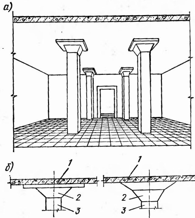
Рис. 110. Железобетонное монолитное безбалочное перекрытие: а — общий вид; б — схема опирания плиты на колонну; 1 — плита; 2 — капитель; 3 — колонна
