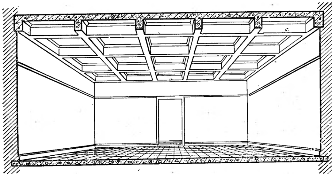
Рис. 109. Общий вид железобетонного монолитного кессонного перекрытия
