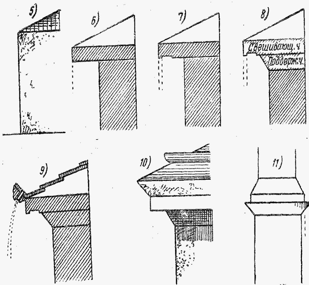
Рис. 5 — 11. Элементы карниза
