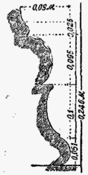
Угловая капитель
