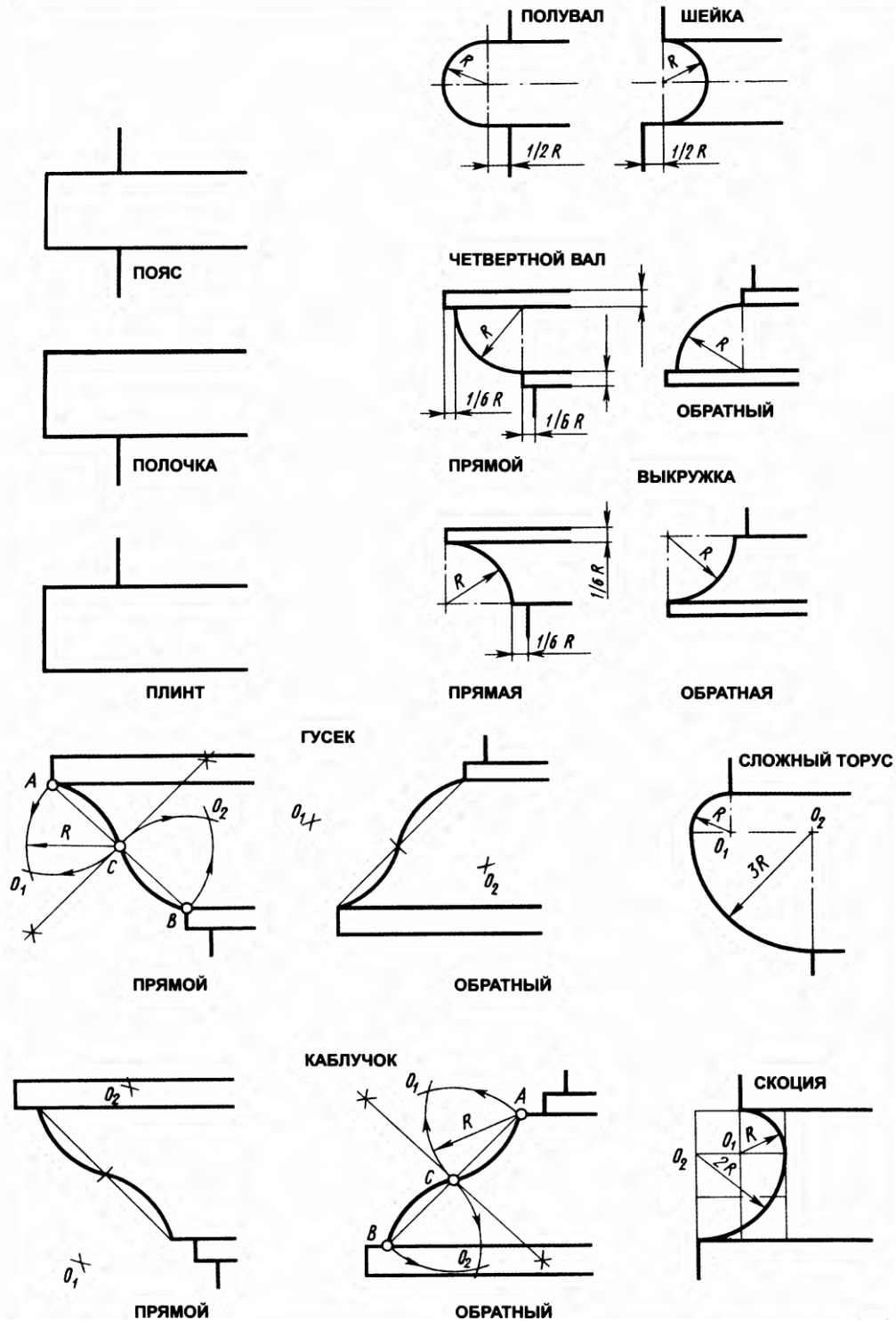
Рис. 1.1. Архитектурные обломы
