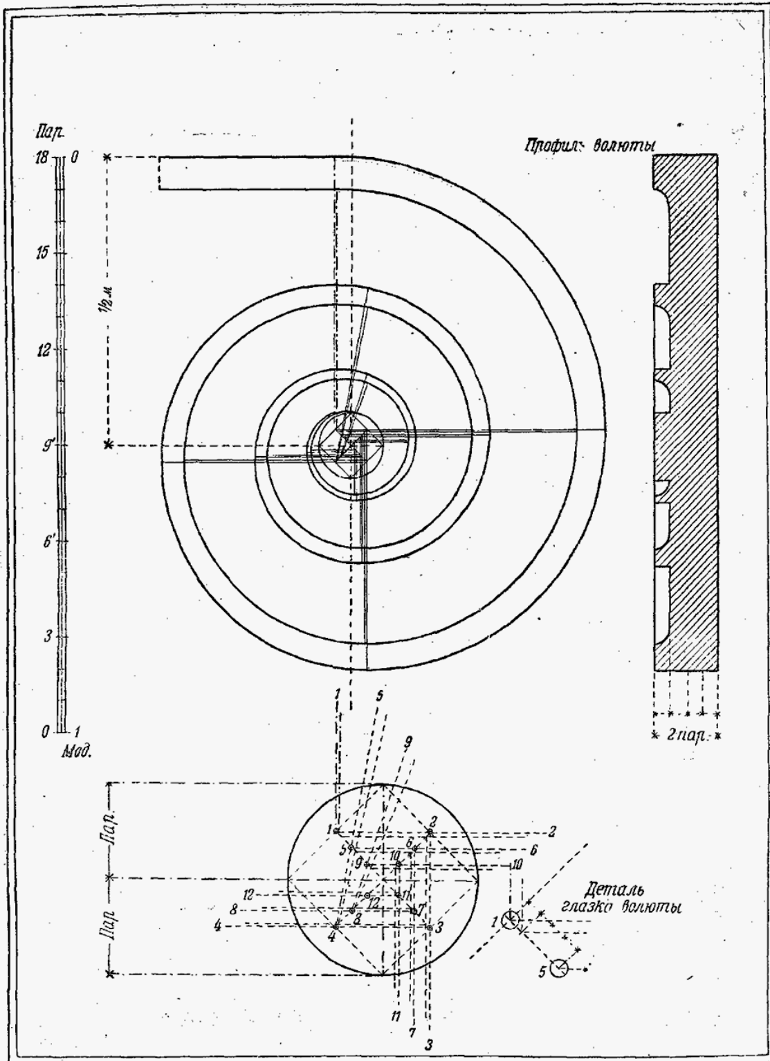
Построение волуты ионической капители
