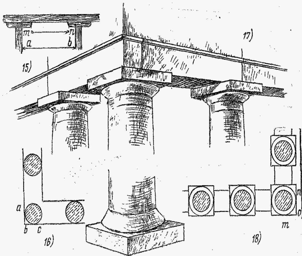
Рис. 15—18. Свес архитрава и капители
