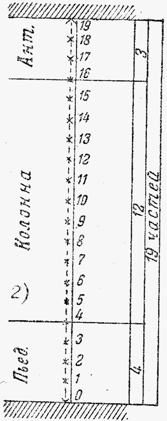
Рис. 1-2. Соотношение главных частей ордера
